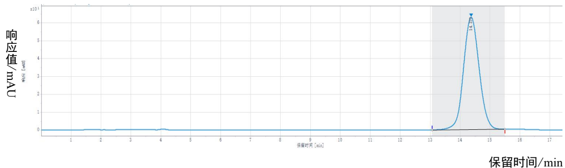
图 C.1 胍基乙酸标准溶液 (50 µg/mL) 的高效液相色谱图
