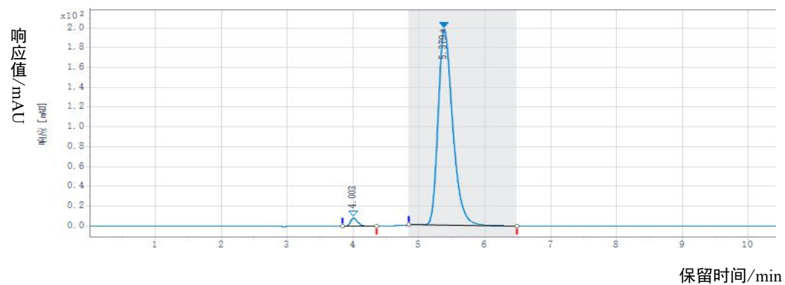
图 C.2 单氰胺、双氰胺混合标准溶液 (40 µg/mL) 的高效液相色谱图
