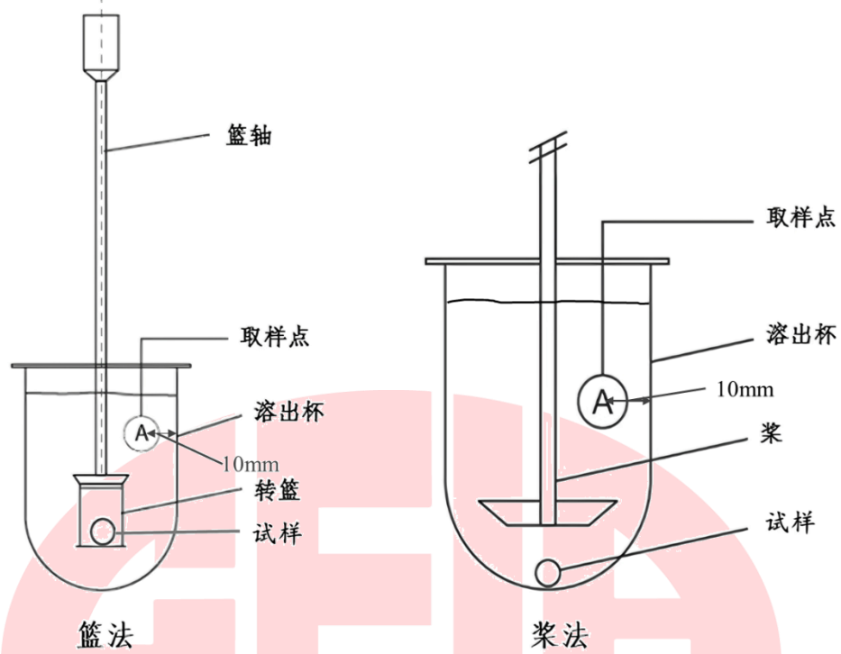
图 B.1 释放度测定篮法（左）和浆法（右）装置示意图
