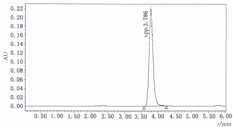
图 A.1 烟酸标准溶液(15 µg/mL) 色谱图
