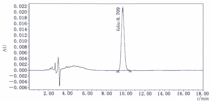
图 A.2 叶酸标准溶液(6 µg/mL) 色谱图
